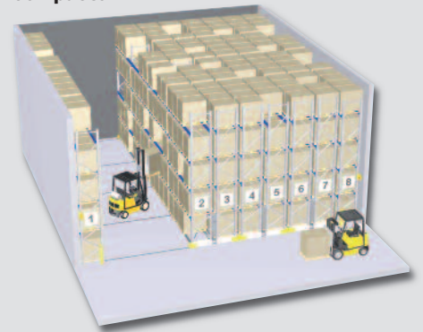
Sistemas móviles de almacenamiento compacto
